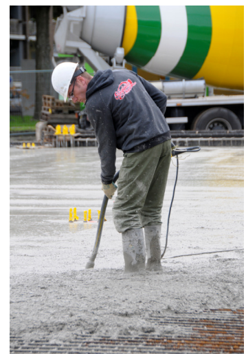
Afbeelding 3. De vloer van de aardwarmtecentrale wordt gestort.
